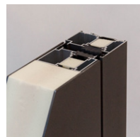
Aluminiowe skrzydło drzwiowe i ościeżnica
