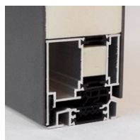
Skrzydło aluminiowe z 4-stronną przylgą
