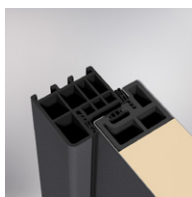
Skrzydło drzwiowe z ramą absiglass
