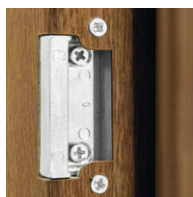
Regulacja języka
