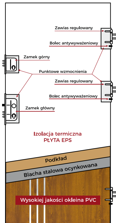
DRZWI STALOWE
