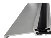
Próg aluminiowy z przekładką termiczną
