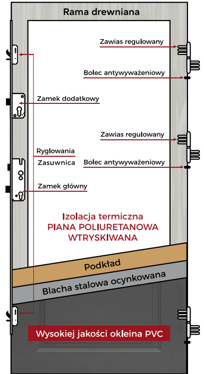
DRZWI HYBRYDOWE NA OŚCIEŻNICY AbsiglassJ
