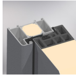
Ościeżnica aluminiowa z wkładem termicznym
