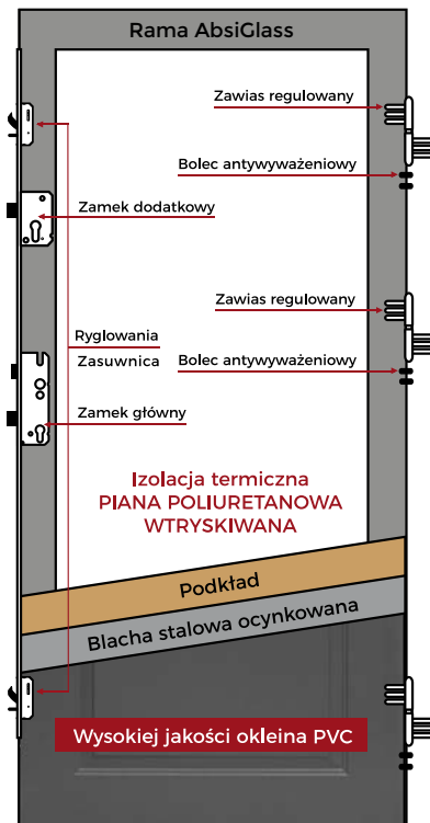
DRZWI PASYWNE NA OŚCIEŻNICY AbsiGlass
