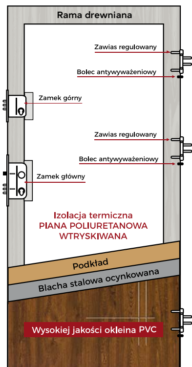
DRZWI STALOWE
