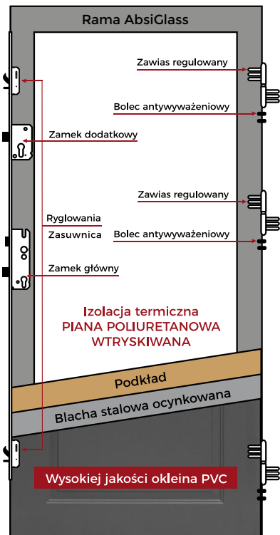
DRZWI PASYWNE NA OŚCIEŻNICY ALUMINOWEJ
