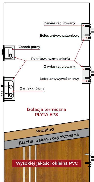
DRZWI STALOWE
