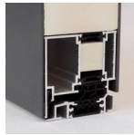
Skrzydło aluminiowe z 4-stronną przylgą
