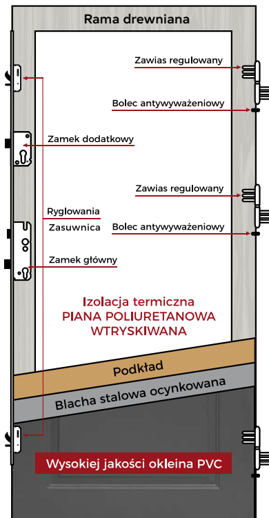
DRZWI HYBRYDOWE NA OŚCIEŻNICY AbsiGlass
