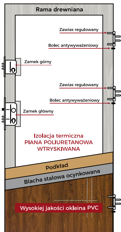
DRZWI STALOWE
