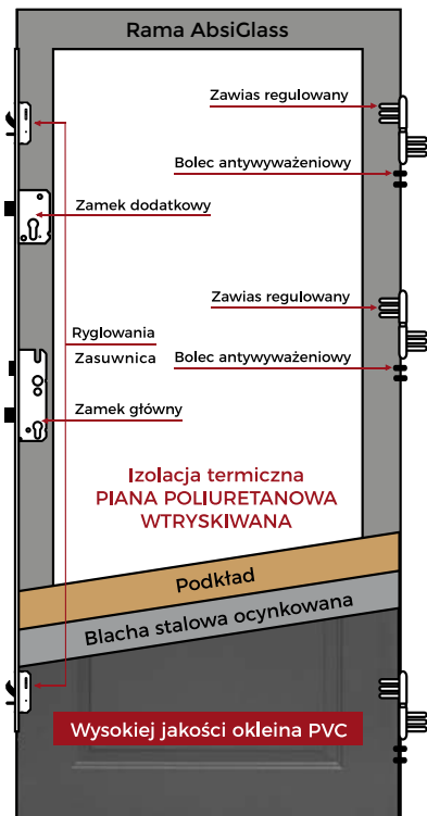
DRZWI PASYWNE NA OŚCIEŻNICY ALUMINIOWEJ
